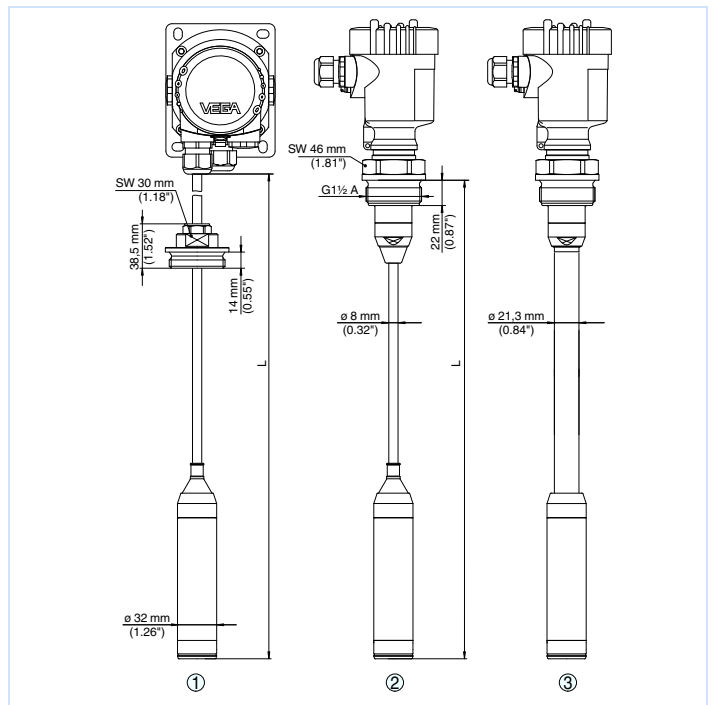
Размеры VEGABAR 66
