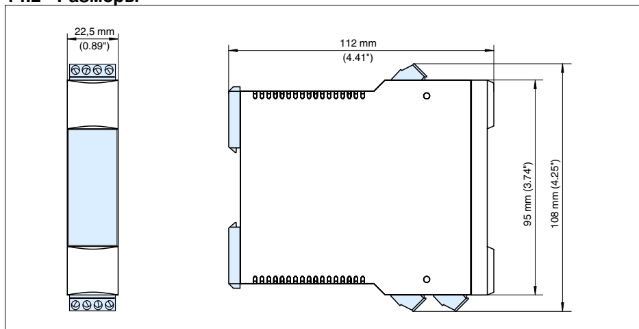
Рис. 141: Размеры VEGATOR 632
