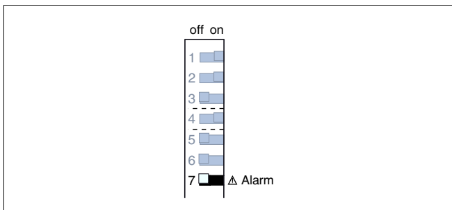
Рис. 99: Блок переключателей (А) с переключателем (7) для активирования контроля обрыва линии (тревожного сигнала)
