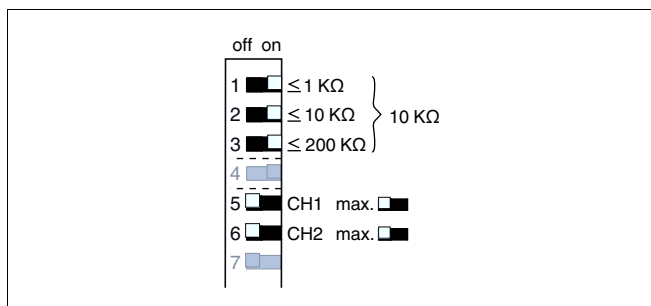
Рис. 96: Диапазон сопротивления до 10\text{ k}\Omega
